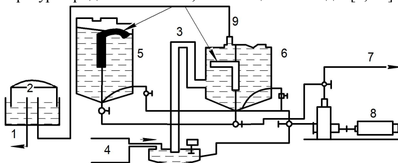
Рис. 1.4 Система Шмідта-Егергюса.
