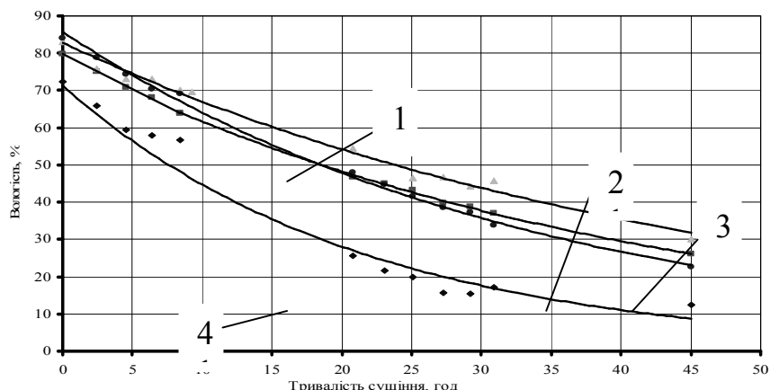
Рис. 2. Динаміка вологовіддачі вегетативними органами плющеної люцерни (фаза бутонізації - початок цвітіння): 1 – третина верхньої частини стебла; 2 – листки; 3 – ціла рослина; 4 - нижня третина стебла (умови проведення дослідів: температура повітря в приміщенні 22 – 23 0 С; відносна вологість повітря 50 – 55 %).
