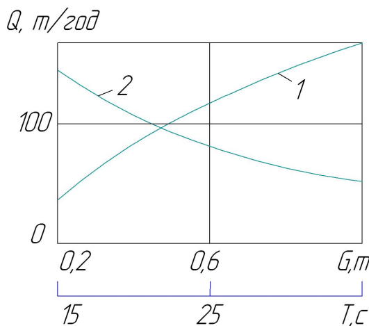
Рис. 6. Залежність продуктивності Q навантажувача від маси G разової блок-порції консервованого корму і часу циклу T .
