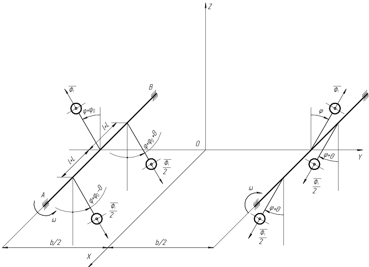
Рис. 1. Расчетная схема блока управляемых вибровозбудителей
