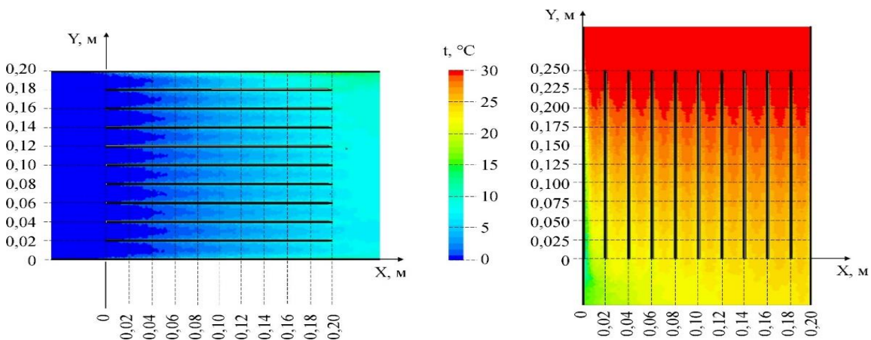
Рис. 8. Повздовжній розподіл температурного поля в теплообміннику побічно-випарного із квадратними каналами
