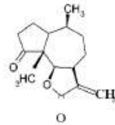
Дамсін
