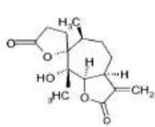
Псилостахіїн
