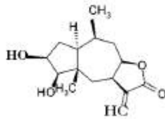
Куманін
