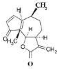
Амброзін
