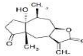
Перувін
