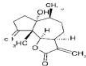
Коронопілін
