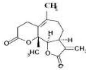
Псилостахіїн В
