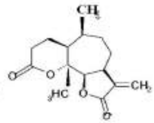
Псилостахіїн С
