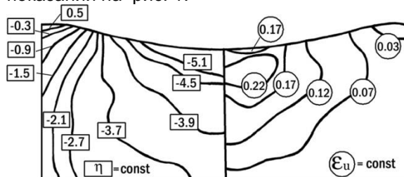
Рис. 1. Розподіл в зоні пластичного відбитку ізоліній: \eta = const (□) і \varepsilon_u = const (○)
