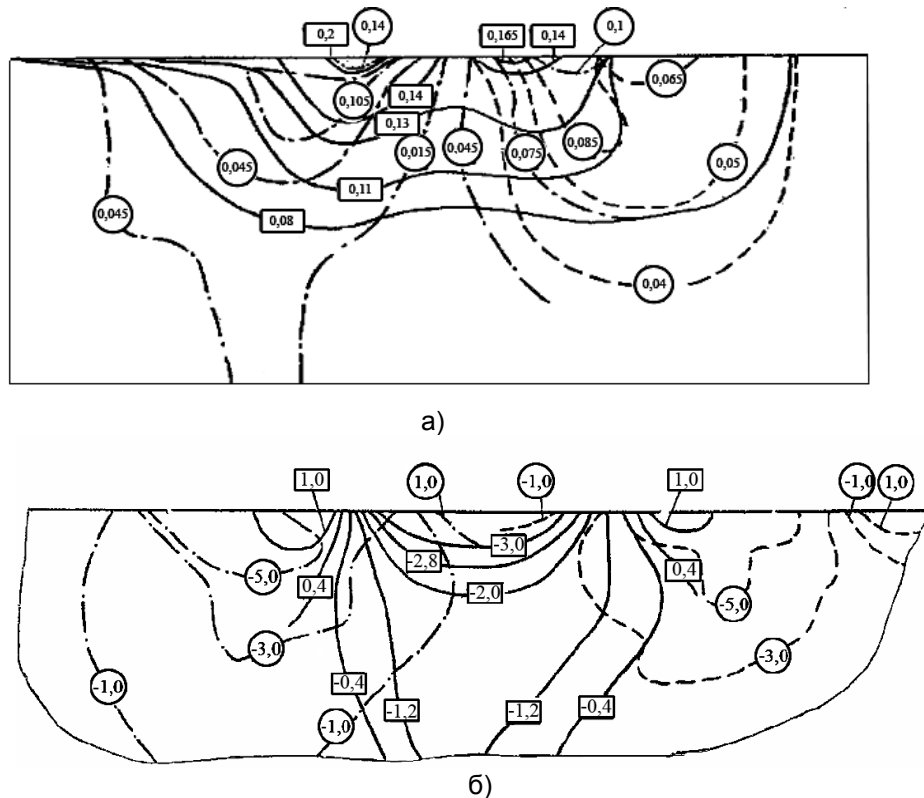
Рис. 2. Характер розподілу інтенсивності деформацій \epsilon_u = const а) і показника напруженого стану \eta = const б) при трьохкратному втискуванні ролика діаметром 12 мм (ширина відбитка 2,5 мм, відстань між першим і другим відбитками 2 мм), після втискування: --- першого; - . - . - . другого; _____ третього.
