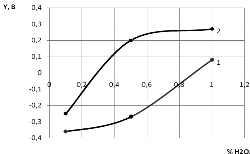
Рис. 1. Влияние добавок H_2O_2 (30%) в 1% растворе HNO_3 на величину потенциала при вибрационной обработке: 1 – сталь 40; 2 – сталь 12X18H10T
