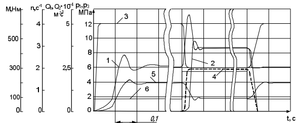
Рис. 6. Теоретичні залежності p_1(t) , p_3(t) , Q_1(t) , Q_2(t) , n(t) , M(t) (криві 1, 2, 3, 4, 5, 6 відповідно) за p_{ке}=12 МПа, крутильної жорсткості c_\phi=0,37 \cdot 10^{-3} Н·м/рад; f_3/f_4=0,63 та ступінчастої зміни навантаження
