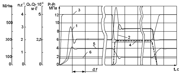
Рис. 3. Теоретичні залежності p_1(t) , p_3(t) , Q_1(t) , Q_2(t) , n(t) , M(t) (криві 1, 2, 3, 4, 5, 6 відповідно) за p_{ке}=12 МПа, крутильної жорсткості 3c_\phi=1,11 \cdot 10^{-3} Н·м/рад; f_3/f_4=0,6 та ступінчастої зміни навантаження
