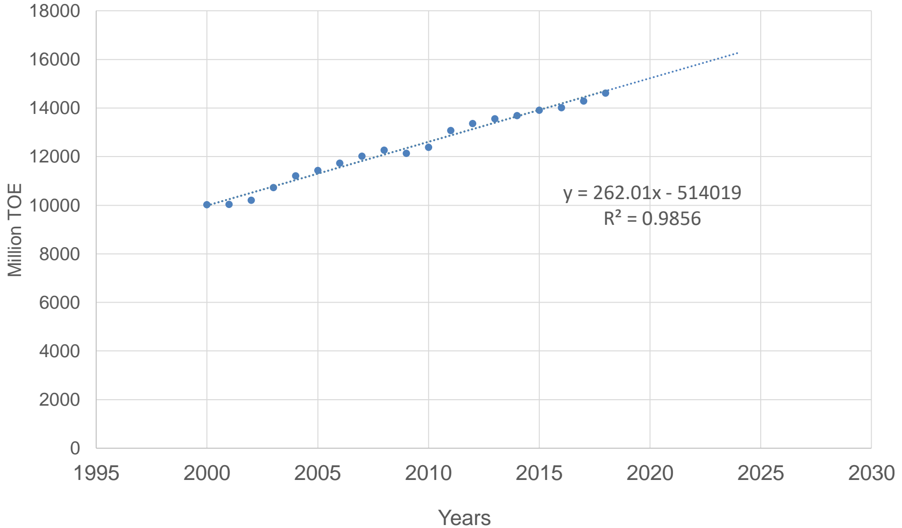
Рис. 1. Лінія тренду загального світового споживання різних видів первинної енергії
