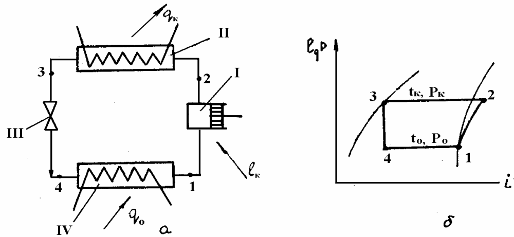
Рис. 5. Схема циклу теплового насосу (а) і побудова його процесів в діаграмі \lg P - I (б): I – компресор. II – конденсатор. III – регулюючий вентиль. IV – випарник. 1 – 2 – адіабатичне стиснення робочого середовища в компресорі; 2 – 3 – конденсація робочої речовини в конденсаторі; 3 – 4 – ізоентальпійне розширення робочої речовини в регулюючому вентилі; 4-1 – ізобарне кипіння робочої речовини у випарнику
