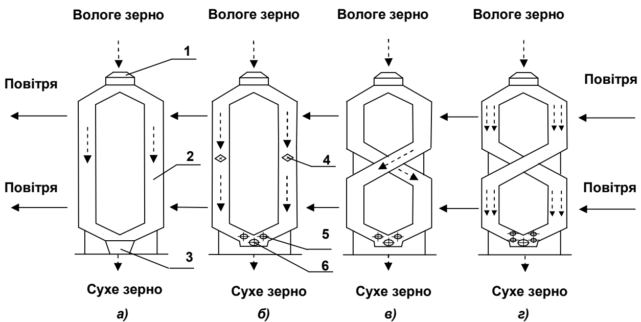
Рис. 3. Схеми вивантаження зерна з колонкових сушарок: а) з простим вивантаженням зерна; б) з інвенторами для перемішування зерна і двома дозуючими валками; в) з хрестовидним рухом зерна і з двома дозуючими валками; г) з хрестовидним рухом зерна і з чотирма дозуючими валками
