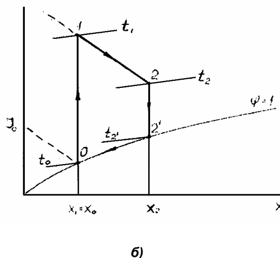
Рис. 7. Схема сушильної теплонасосної установки з повним поверненням відпрацьованого сушильного агента (а) та діаграма I – x (б): I – калорифер(конденсатор); II – сушильна камера; III – охолоджувач(випарник); IV – сепаратор; V – дросельний вентиль; VI – турбокомпресор. 0 – 1 – нагрівання в калорифері; 1 – 2 – сушіння в сушильній камері; 2 – 2' – охолодження до лінії насичення; 2' – 0 – кінцеве охолодження на лінії насичення
