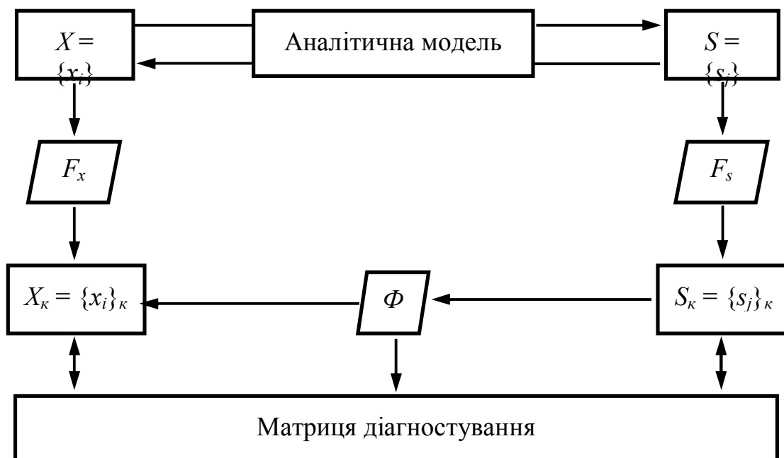
Рис 2. Блок-схема синтезу матриці діагностування: X = \{x_i\} – нескінченна кількість технічних станів об'єкта; X_k = \{x_{i,k}\} – кінцева кількість технічних станів; S = \{s_j\} – нескінченна множина ознак технічних станів об'єкта;
