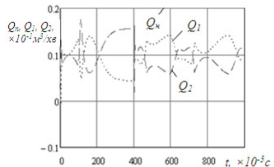
Рисунок 5 — Перехідний процес в системі гідроприводів при настройці упора b_2 = 4 \text{ мм} , діаметра золотника d_{зол} = 19,5 \text{ мм} , жорсткості пружини C_{пр} = 0,3 \text{ Н}/\text{мм}
