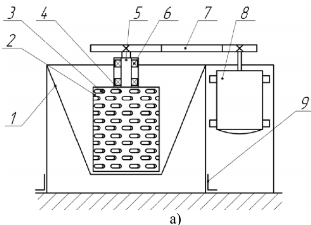
Рис. 2. Подрібнювач коренеплодів: а) схема подрібнювача б) загальний вигляд
